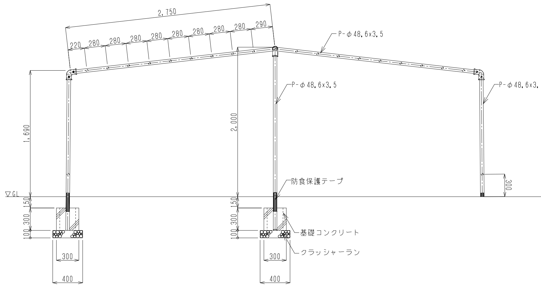
正面図
