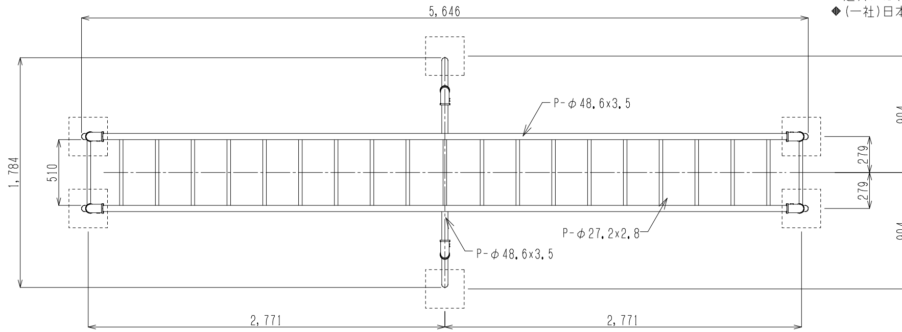
平面図
