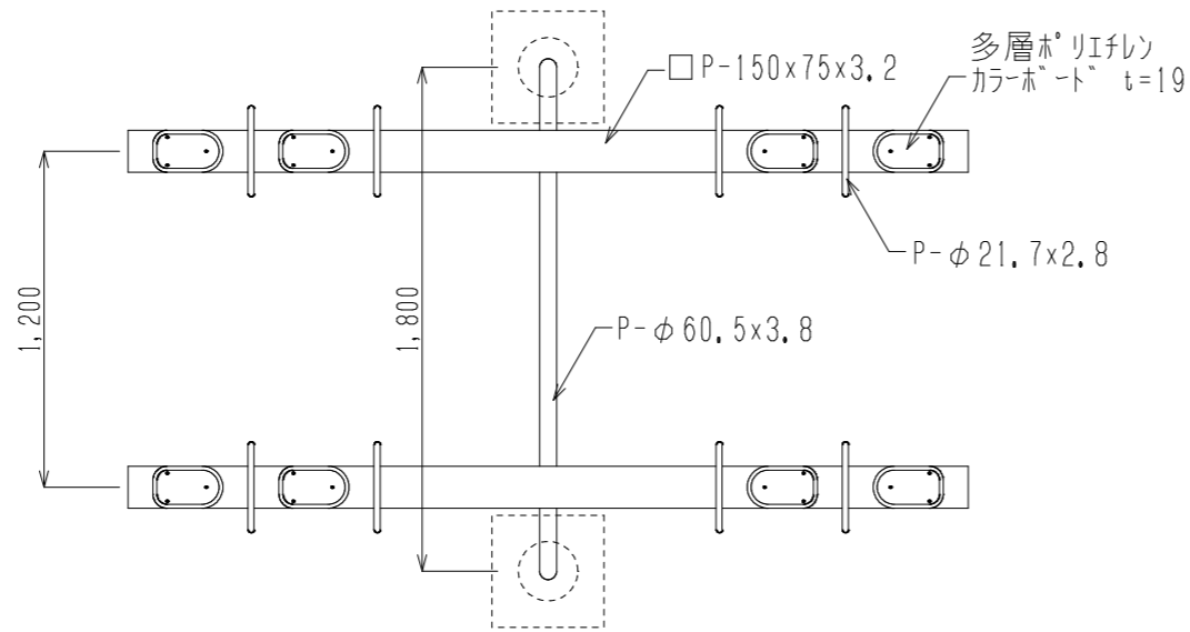
平面図
