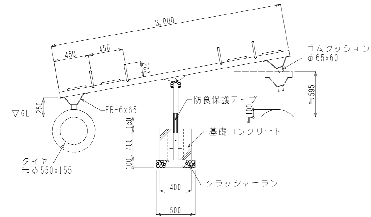
正面図
